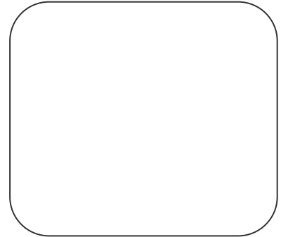
円柱
