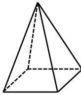
四角錐
